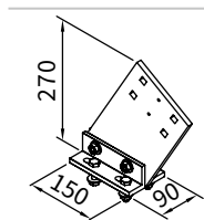
Wspornik krokwiowy
