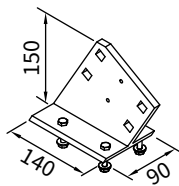
Wspornik krokwiowy
