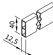
Listwa dystansowa do profilu łączenia ściennego
