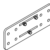
Płyta mocująca A 430 × 160 × 12 mm
