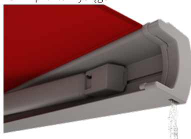
3 Specjalny odpływ wody w profilu wysięgu
