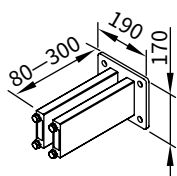
Wspornik dystansowy do uchwytu ściennego 300 mm 75877. i 75878.
