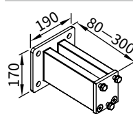
Wspornik dystansowy do uchwytu ściennego 100 mm 75885. i 75886.
