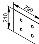
Błacha osłonowa do płyty dystansowej i wspornika dystansowego 77968. przy tynku izolacyjnym 290 x 210 x 2 mm
