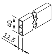
Listwa dystansowa do profilu łączenia ściennego towar z metra
