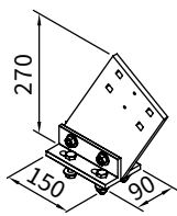
Wspornik krokwiowy
