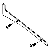
1 blacha boczna łącznie z 2 blachowkrętami z łbem soczewkowym do profilu przyłącza ściennego
